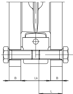
LUGGED
