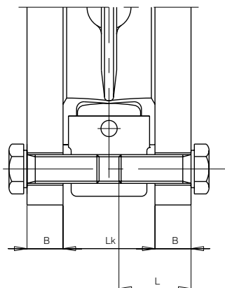
LUGGED
